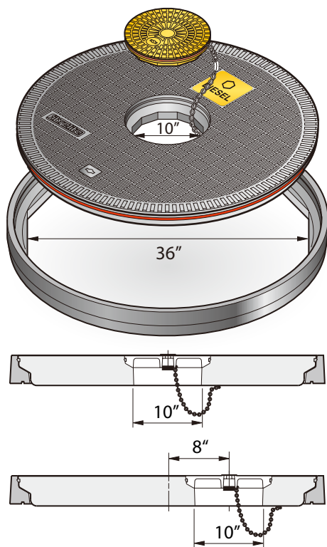
FL90 - 36" dia. Fill Covers
