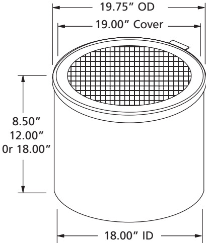
18" MANHOLE
